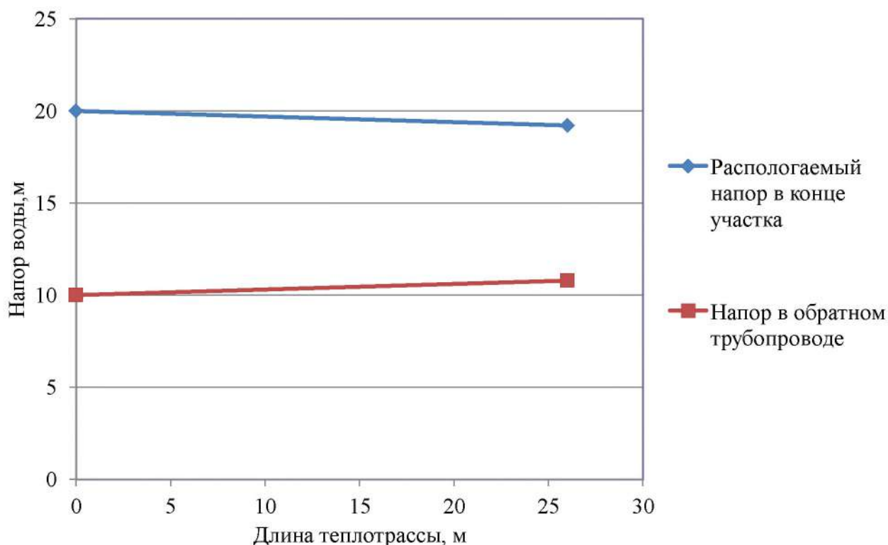
Рисунок 2.4 – Пьезометрический график тепловой сети школьной котельной с. Баярак от котельной до школы
