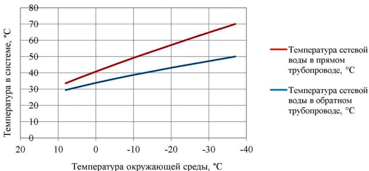
Рисунок 2.3 – График изменения температур теплоносителя 70–50 °С
