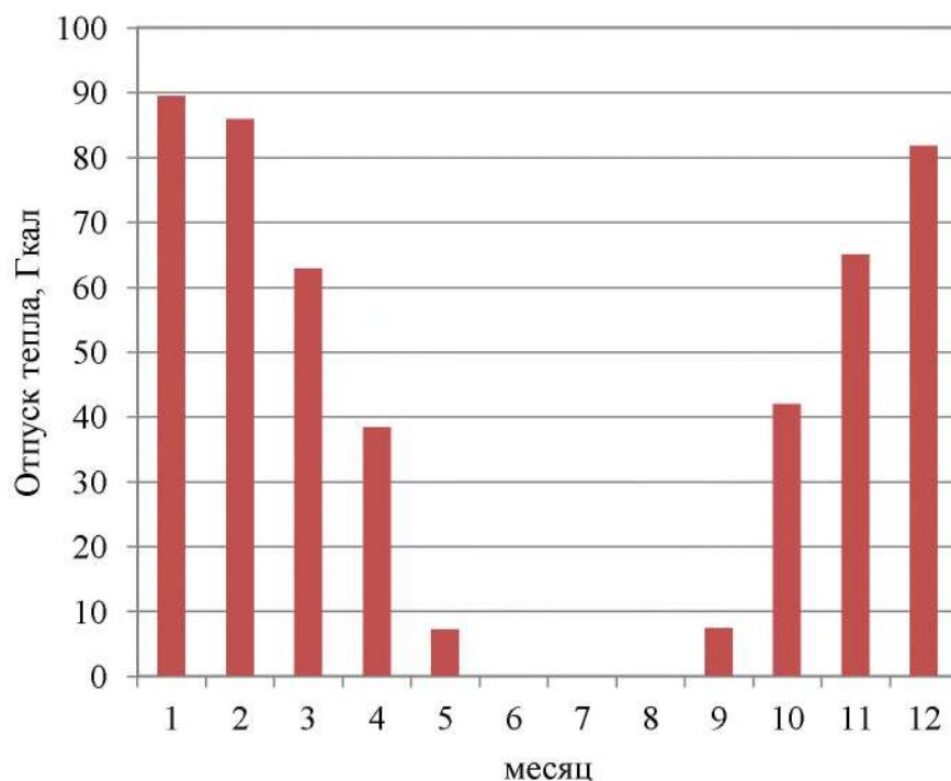
Рисунок 1.3 – Оптимальный температурный график отпуски тепловой энергии для Школьной котельной с. Баярак
