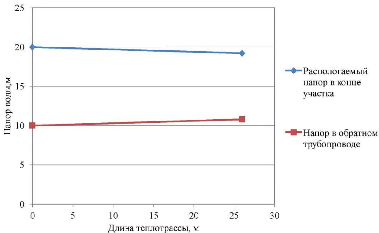
Рисунок 2.5 – Пьезометрический график тепловой сети школьной котельной с. Баярак от котельной до школы
