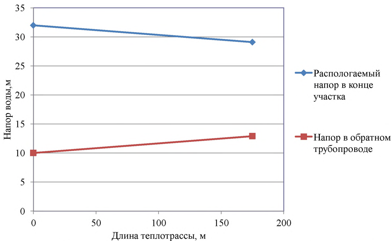
Рисунок 2.5 – Пьезометрический график тепловой сети школьной котельной с. Скаты от котельной до школы
