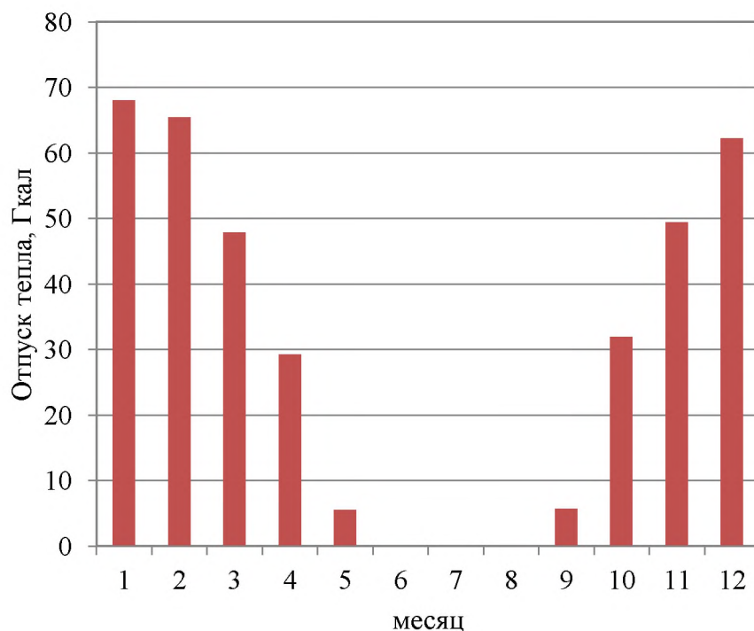
Рисунок 1.3 – Оптимальный температурный график отпуски тепловой энергии для Школьной котельной с. Скаты
