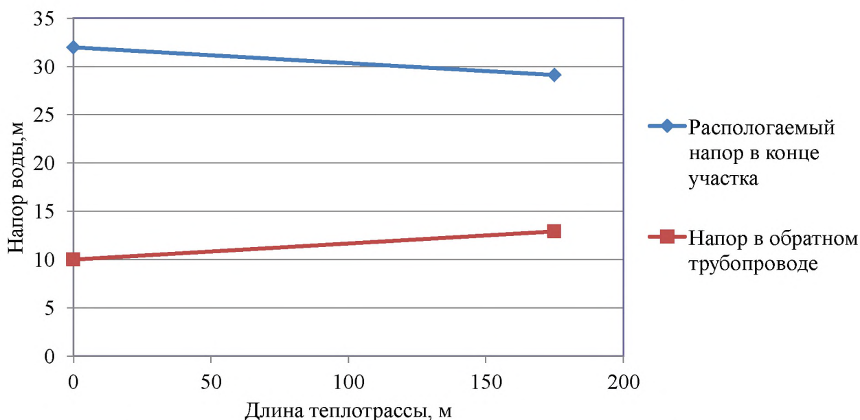
Рисунок 2.4 – Пьезометрический график тепловой сети школьной котельной с. Скаты от котельной до школы
