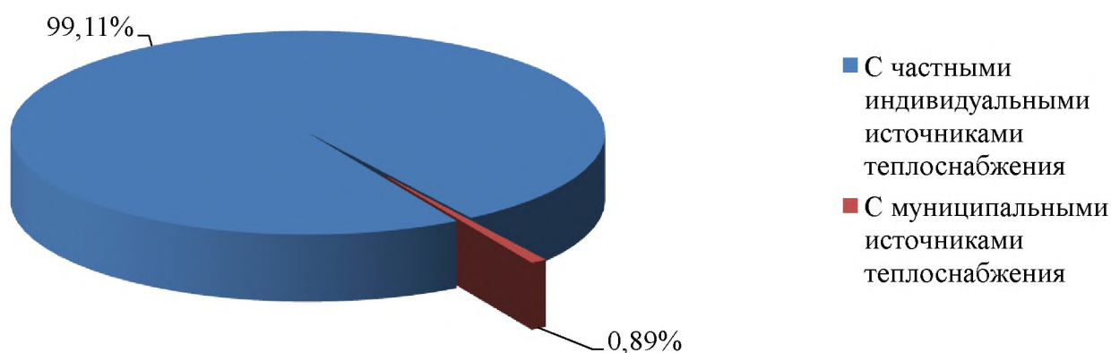
Рисунок 1.2 – Соотношение площади охвата зоны действия с частными индивидуальными и муниципальными источниками тепловой энергии в Скатинском сельсовете
